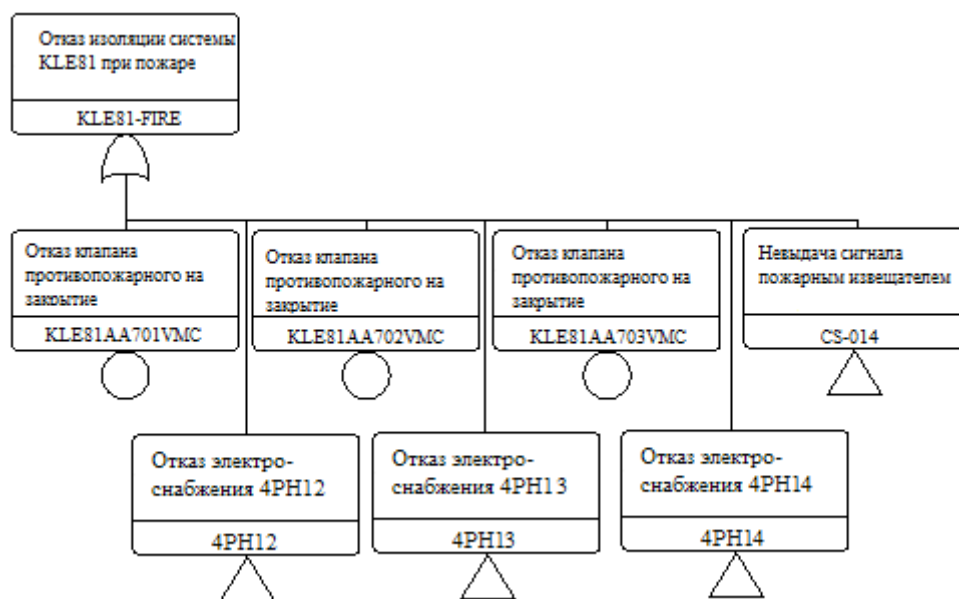
Рис. 4. Дерево отказов «Отказ на изоляцию системы KLE81 при пожаре» (обозначения аналогичны рис. 3)
