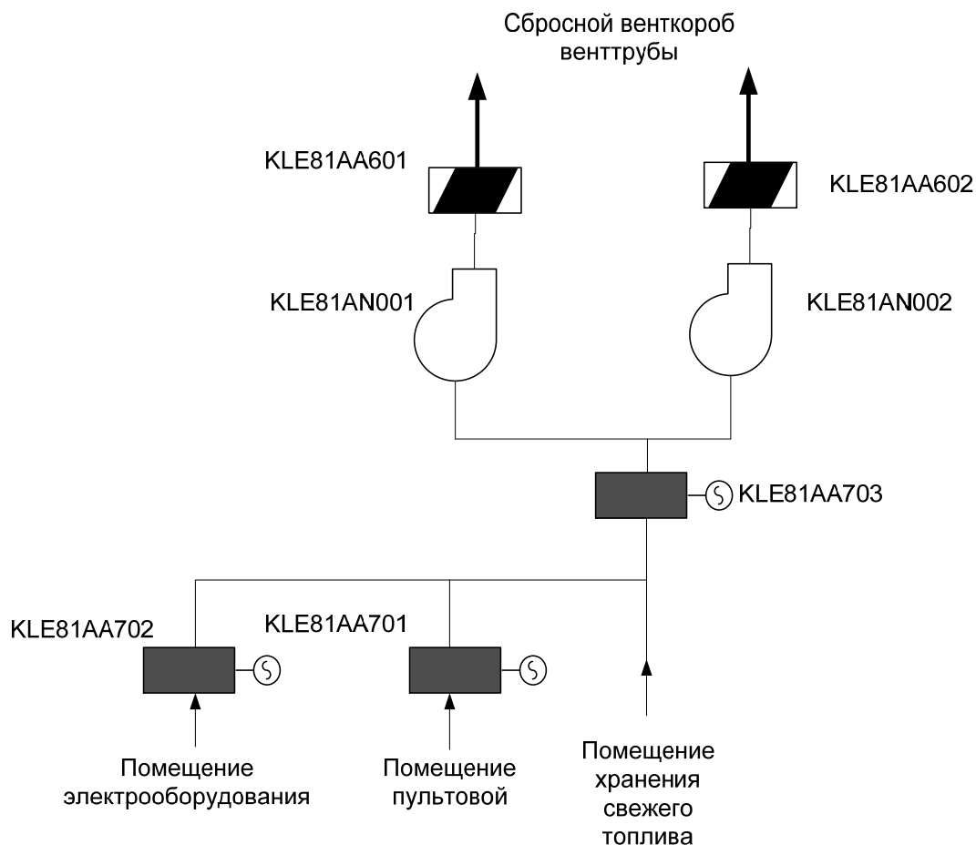
Рис. 2. Упрощенная схема системы вентиляции 4KLE81
