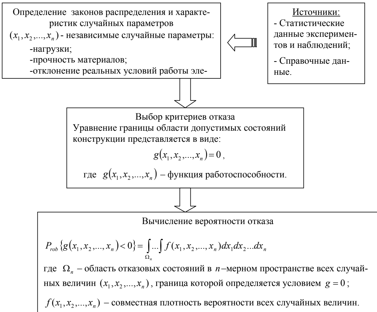
Рис. 1. Схема определения вероятности отказа пассивного элемента
