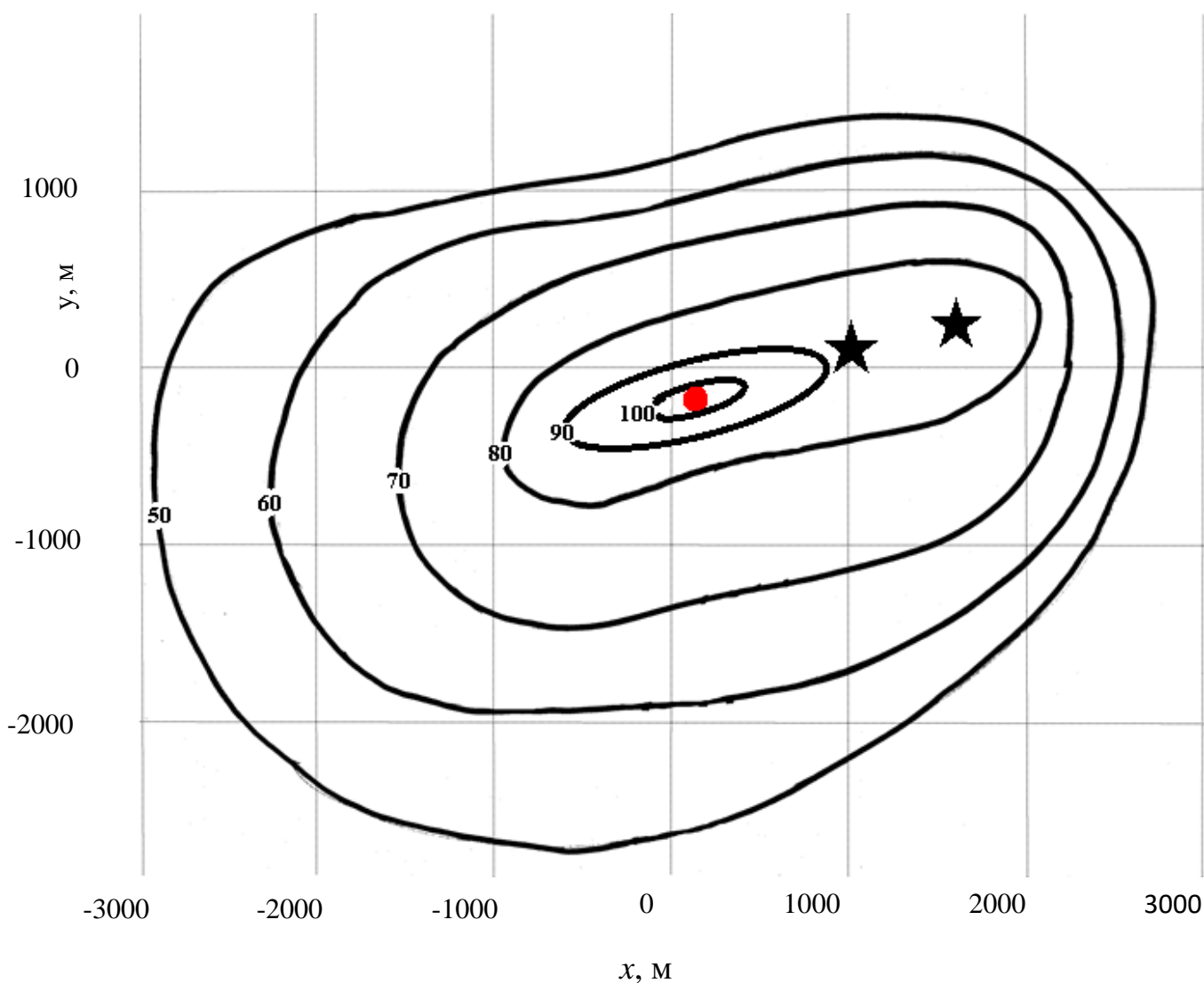
Рис. 3. Рекомендуемый вид графического отображения распределения доз облучения населения в районе расположения организации, осуществляющей выбросы радиоактивных веществ, в виде карты изолиний. Обозначения: ★ — источники выбросов; ● — критическая точка местности
