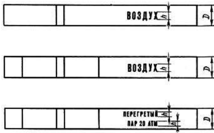
Рисунок 3. Высота маркировочных надписей на трубопроводах
