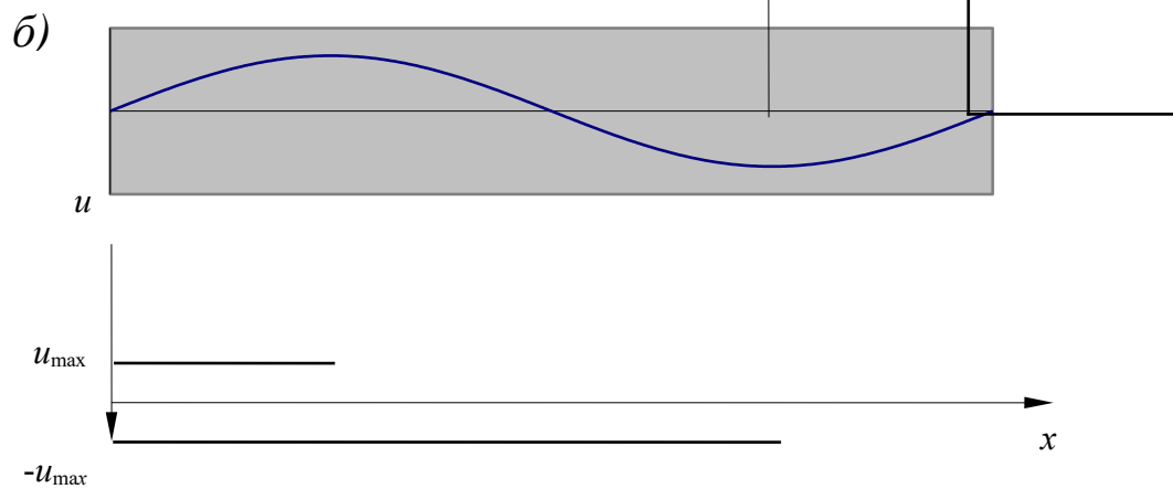
Рис. П.6.1. Деформации линейно-протяженной конструкции при прохождении продольной сейсмической волны: а) – участок подземного трубопровода; б) – перемещения при прохождении продольной волны; a, b – положения узлов трубопровода до деформации; a', b' – то же после деформации
