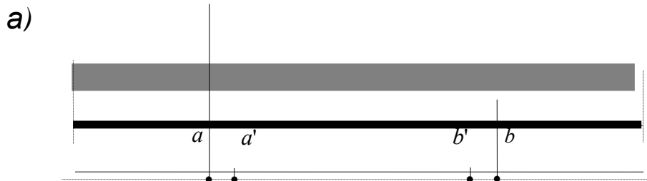
Рис. П.6.1. Деформации линейно-протяженной конструкции при прохождении продольной сейсмической волны: а) – участок подземного трубопровода; б) – перемещения при прохождении продольной волны; a, b – положения узлов трубопровода до деформации; a', b' – то же после деформации
