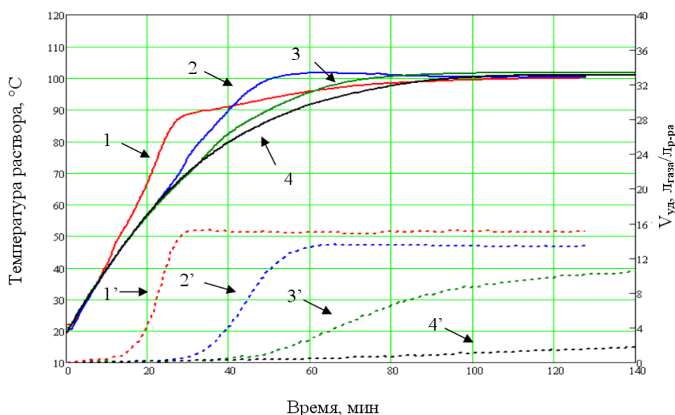
Рис. 2.3.9. Динамики изменения температуры и объема газов при нагревании 0,5 моль/л растворов нитрата гидразина в \text{HNO}_3 концентрации 12 моль/л (1,1'), 9 моль/л (2,2'), 7 моль/л (3,3') и 4 моль/л (4,4') при температуре термостата 100 °C
