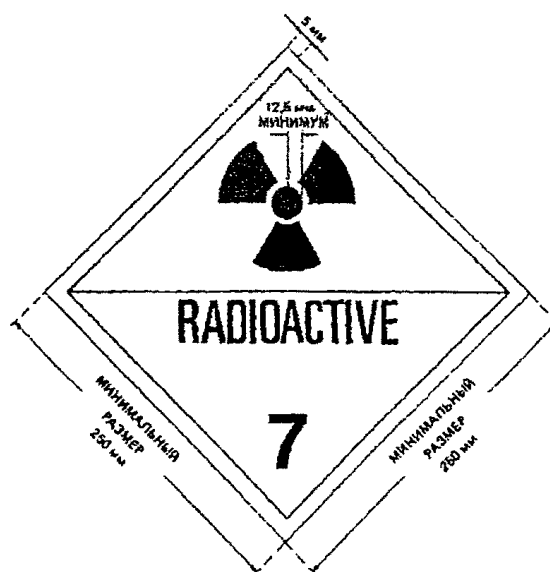
Рис. 5. Информационное табло: указаны минимальные размеры, при использовании больших размеров следует сохранять указанные пропорции; высота цифры "7" должна быть не менее 25 мм; цвет фона верхней половины табло - желтый; нижней половины - белый; цвет основного знака радиационной опасности (трилистника) и надписи - черный; использование слова "РАДИОАКТИВНО" в нижней части необязательно, что позволяет применять это табло для изображения соответствующего номера ООН для груза
