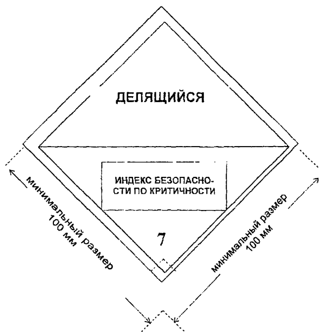
Рис. 5. Этикетка с указанием ИБК: указаны минимальные размеры, при использовании больших размеров следует сохранять указанные пропорции; цвет фона табло - белый; цвет надписей - черный
