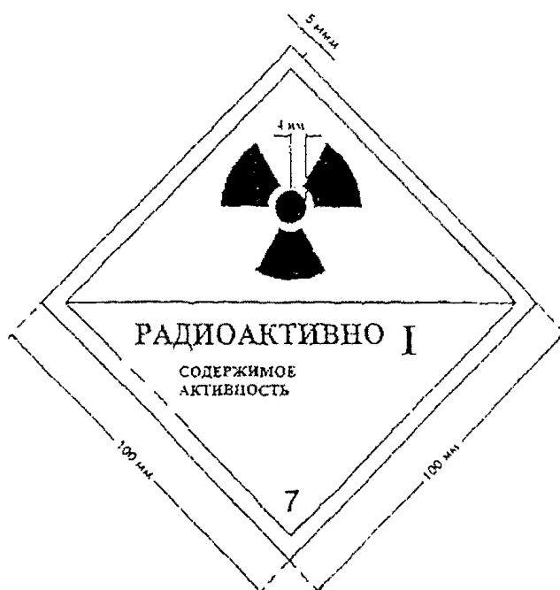
Рис. 2. Этикетка категории "I-БЕЛАЯ": цвет фона этикетки - белый; цвет основного знака радиационной опасности (трилистника) и надписей - черный; цвет полосы, обозначающей категорию, - красный
